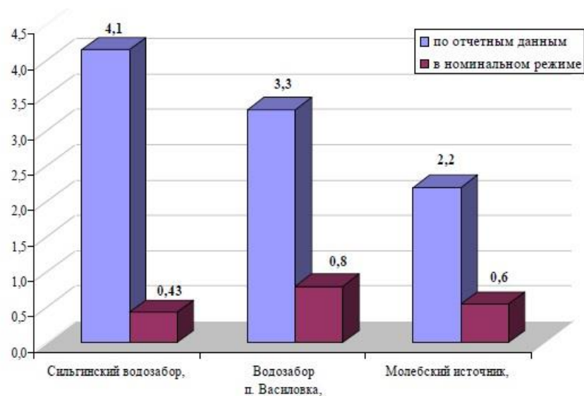
Рис. 6. Сравнение удельного электропотребления на водозаборах по отчетным данным с технической возможностью насосного оборудования.
